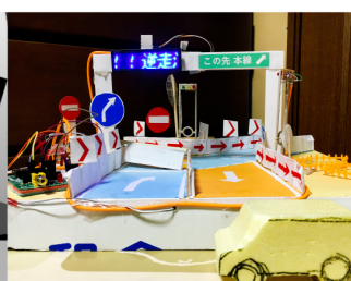
ロボット・電子工作部門 / 小学生の部 逆走防止の交差点 佐藤空汰さん (小学6年生)
